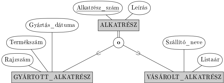
EER diagram egy átfedő (nem diszjunkt) specializáció esetén.
